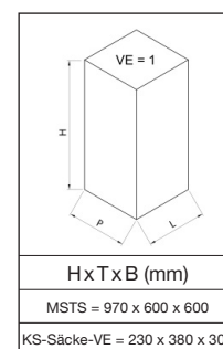
Abb.: MSTS 120, fahrbar, mit Metalldeckel, Art.-Nr. 10281
