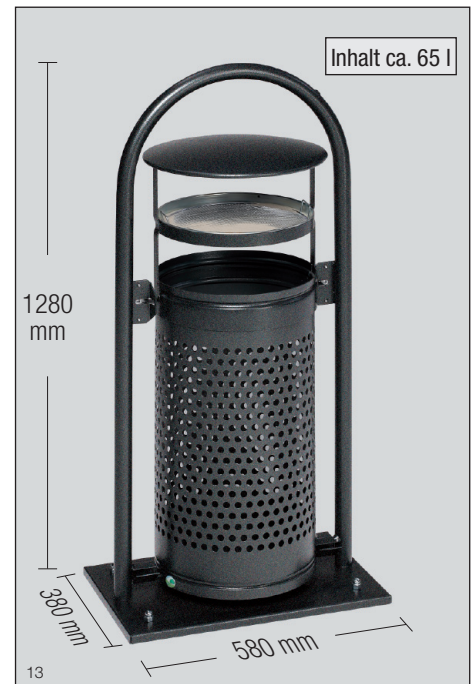
Abb.: Rohrbogenständer RB 002, Art.-Nr. 18714
