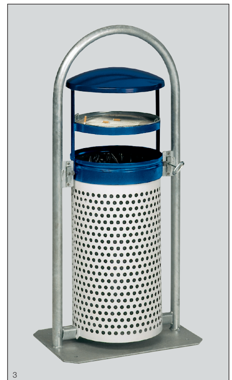
Abb.: Rohrbogenständer RB 002, Art.-Nr. 1870
