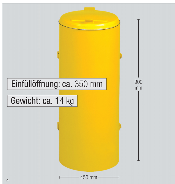
Abb.: Kompakt-Junior mit Einflügeltür, gelb beschichtet, Art.-Nr. 1017
