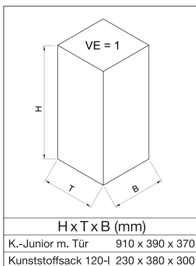
Abb.: Kompakt-Junior mit Einflügeltür, gelb beschichtet, Art.-Nr. 1017
