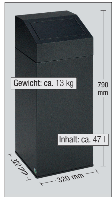
Abb.: Wertstoffsammler 45 l für Metall, Art.-Nr. 12384
