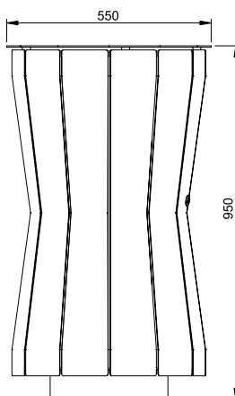
7098 -00 Seitenansicht
