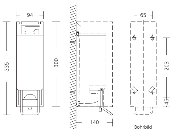
NSU 11 S/D/F Schrankeinbauspender
