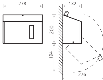
Bohrbild
