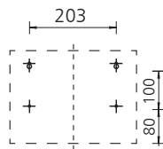
Bohrbild
